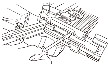
Lame d'entraînement
