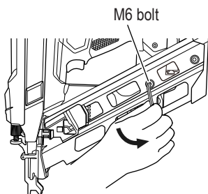
M6 bolt
