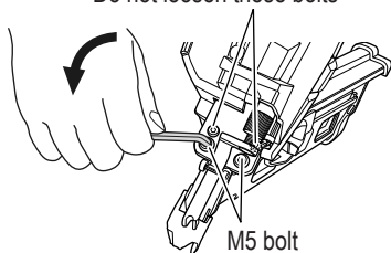
M5 bolt
