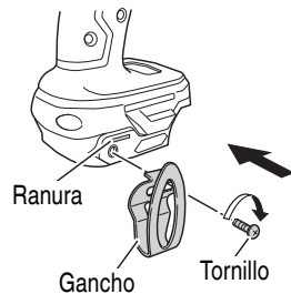
Ranura Gancho Tornillo Fig. 12
